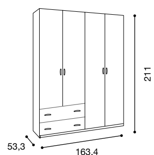
Armadio 4 ante con cassetti
